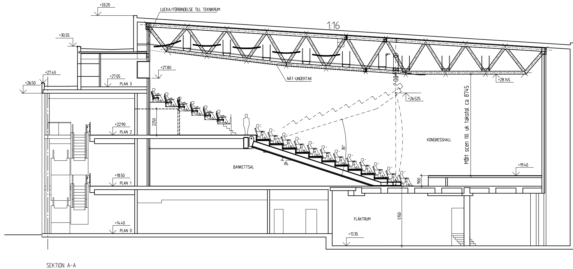
SEKTION A-A
